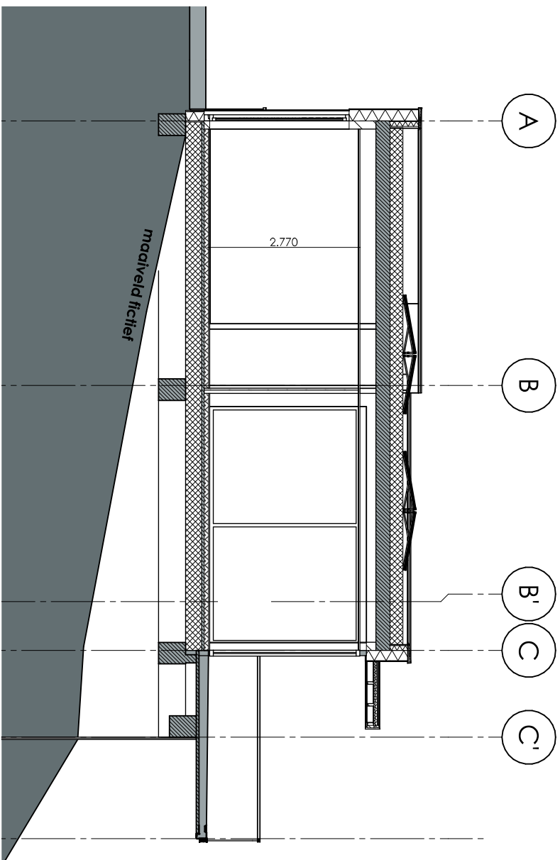
Doorsnede A-A
