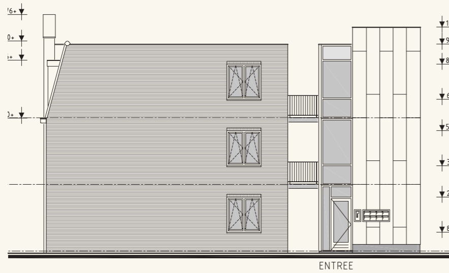
Rechterzijgevel
